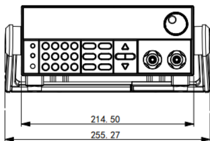
详细尺寸图
