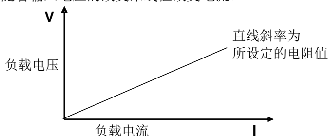
定电阻模式
